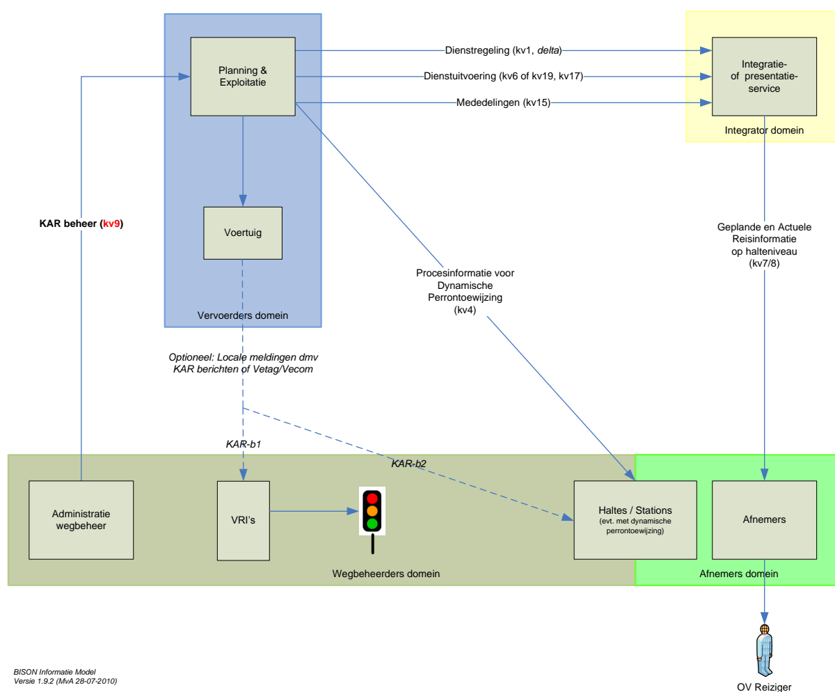
Figuur 1 de BISON architectuur
